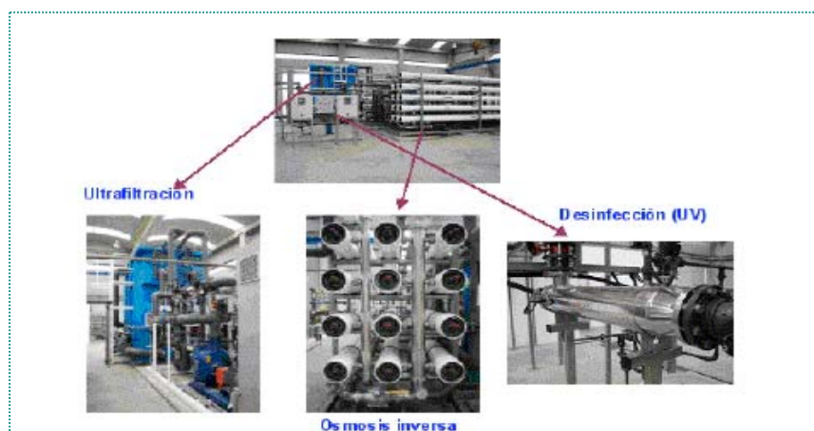
Il·lustració 3: Exemples dels mòduls d'ultrafiltració, osmosis inversa i desinfecció UV per als tractaments d'aigua regenerada en la barrera hidràulica de l'aquífer del Delta de Llobregat.
