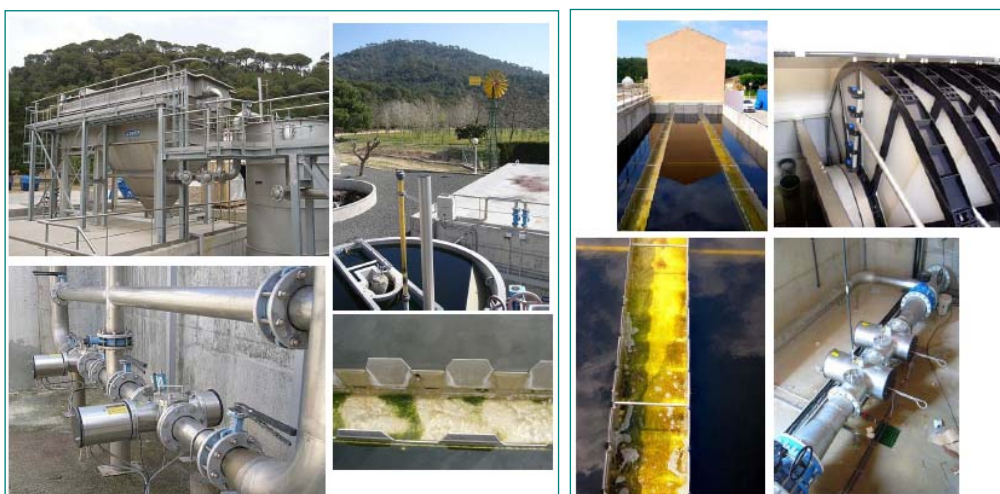
Il·lustració 10: Vistes en detall dels tractaments d'aigua regenerada de L'EDAR a Tossa de Mar.
