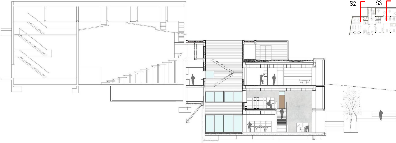
secció S2
