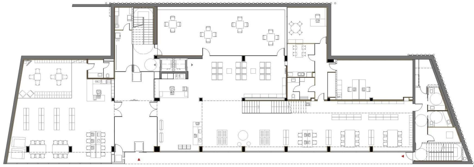
planta baixa
