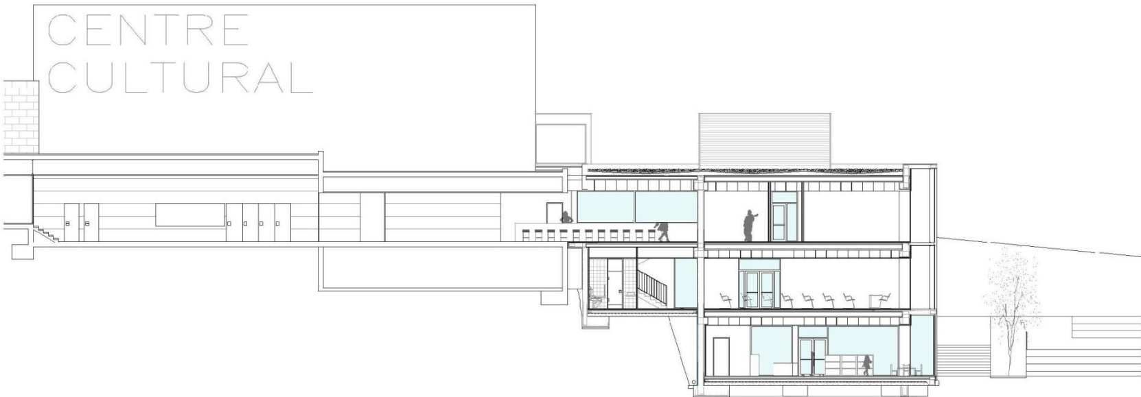
secció S3
