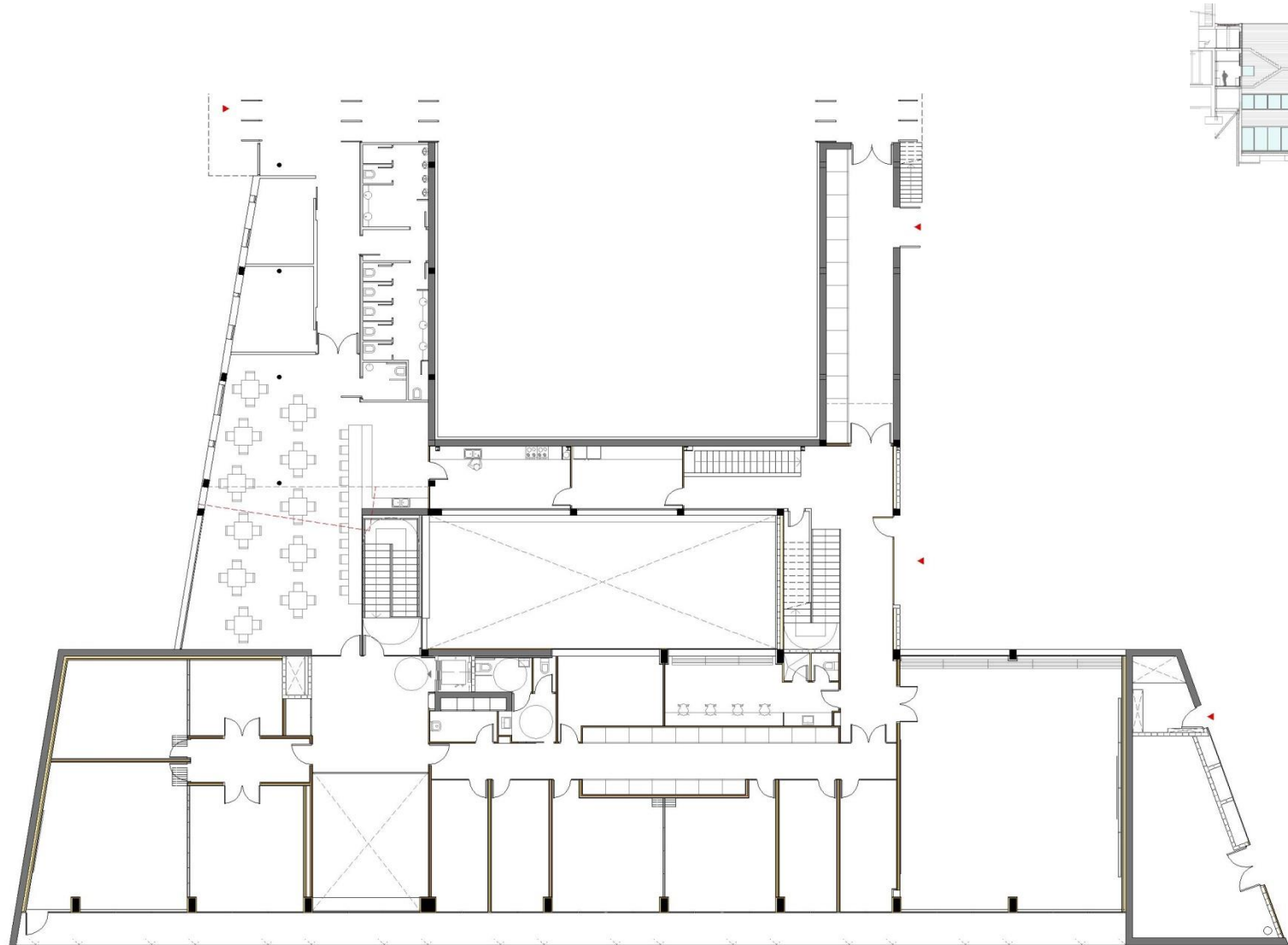
planta segona
