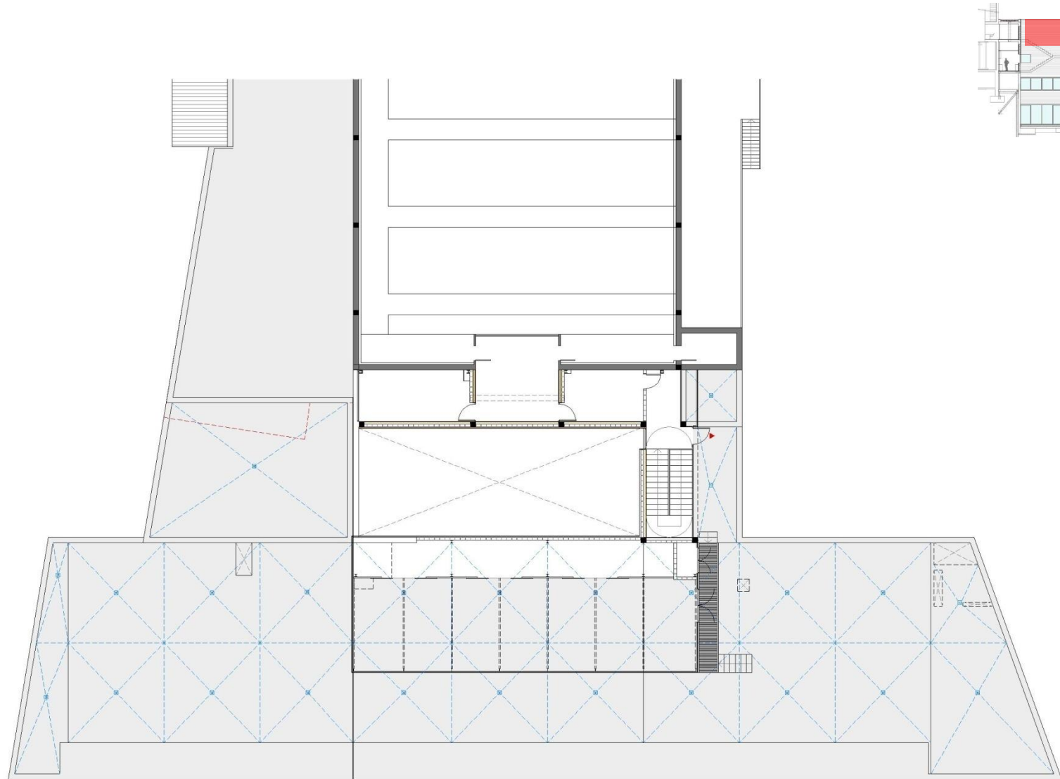
planta coberta
