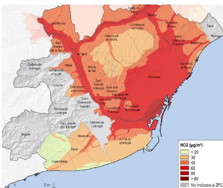
Immissions \text{NO}_2 als municipis AMB que pertanyen la ZPE. Font: Programa metropolità de mesures contra la contaminació atmosfèrica.
