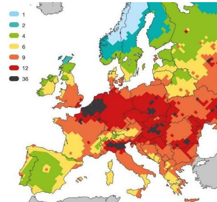
Promig del nombre de mesos que es redueix l'esperança de vida a causa de les partícules ( \text{PM}_{10} o \text{PM}_{2.5} ). Font: Comissió Europea.
