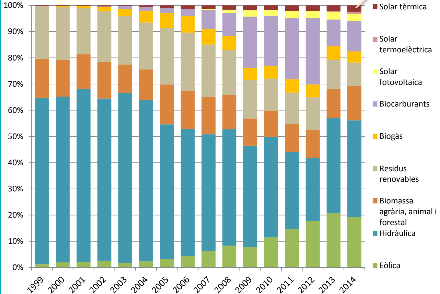
Consum d'energia primària renovable a Catalunya
