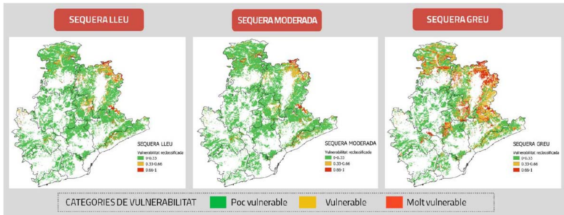
Figura 5: Mapes de la vulnerabilitat predita per categories (baixa entre 0-0.33; mitjana entre 0.33-0.66; i alta entre 0.66-1) segons els escenaris de sequera lleu, moderada i greu per la província de Barcelona, segons el Vulnemap.
